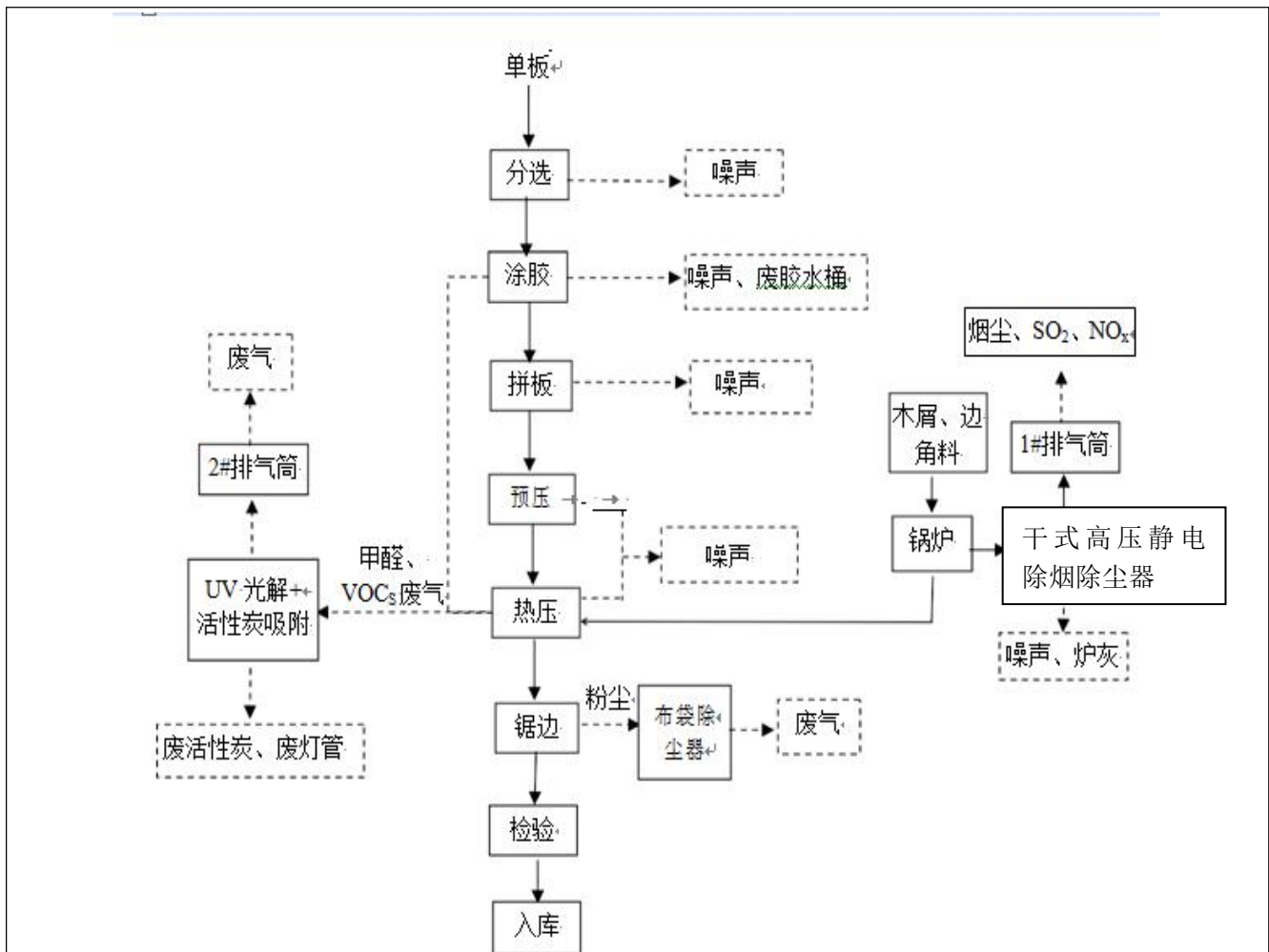
图 2-2 胶合板生产工艺流程图及产污节点图
