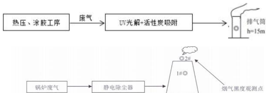
图 3-2 有组织废气监测示意图
