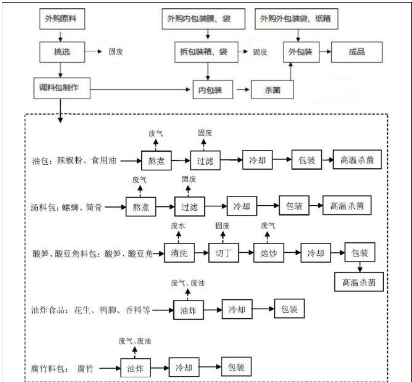
图 2-1 螺蛳粉生产工艺流程图及产污节点图
