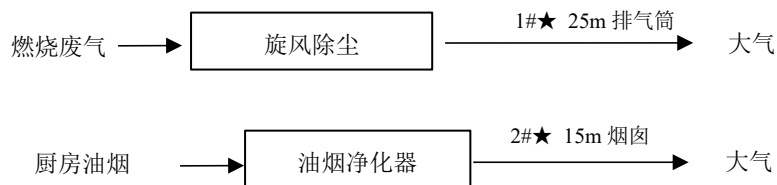
图 3-2 有组织废气处理示意图
