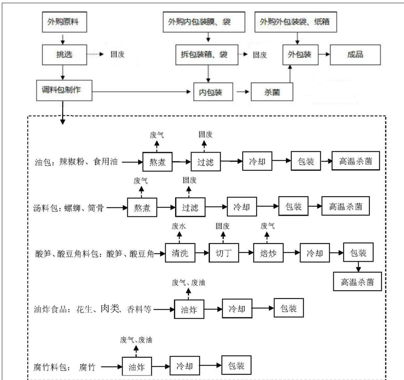
图 2-1 袋装螺蛳粉生产工艺流程图及产污节点图
