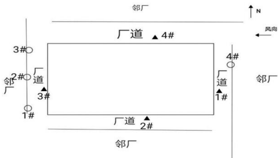
图 3-2 废气处理及监测点位示意图
