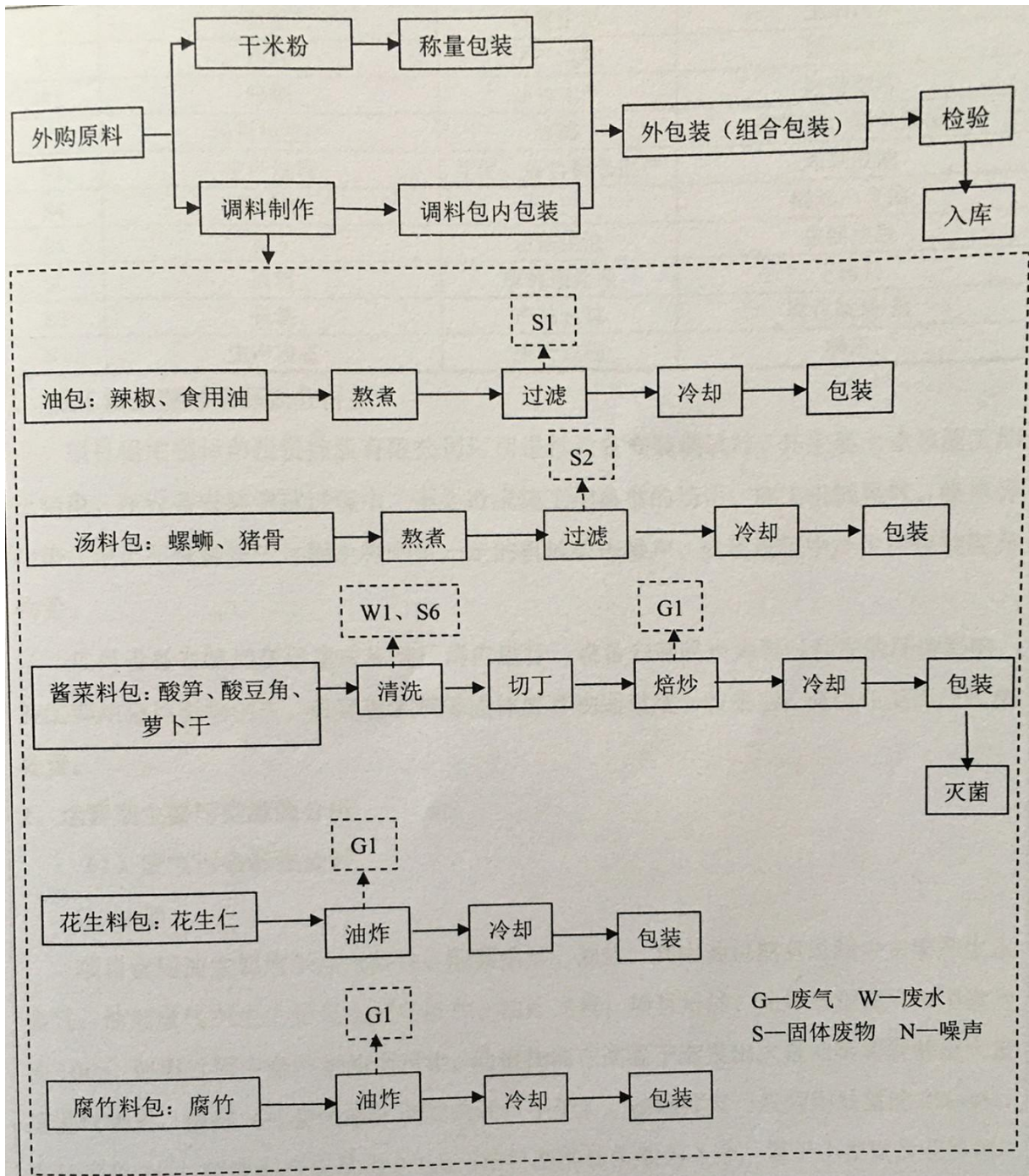
图 2-2 项目生产工艺流程及产污节点图
